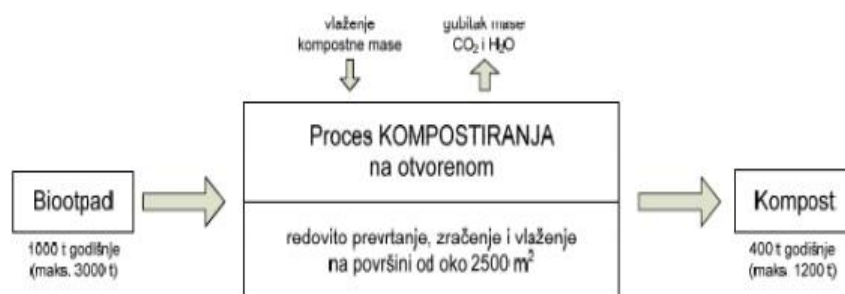
Slika 7: Tehnološka shema procesa kompostiranja
