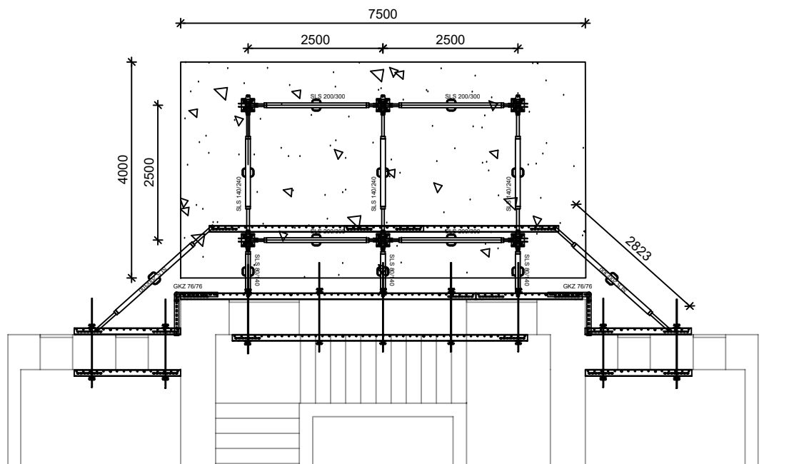
Tlocrt
