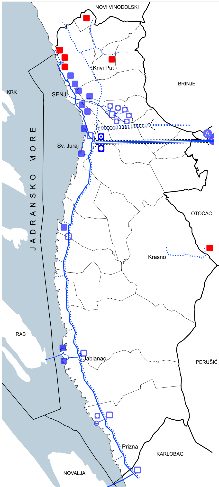
kartogram 3.8. Vodnogospodarski sustav vodoopskrba
